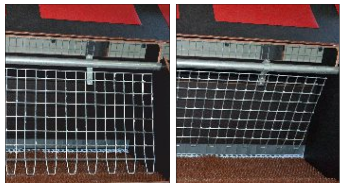
system zamykający otwór gniazda- zamknięty / otwarty
