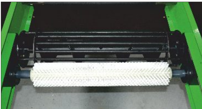
moduł napinania taśmy ze szczotką usuwającą odpady oraz spiralą transportującą odpady poza moduł
